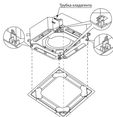
Рисунок 22 - Установка панели
