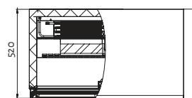
TD103-Bar Глух. дверь TD103-GC
