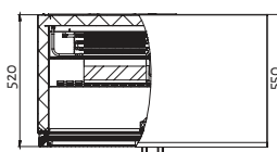
TD102-Bar Глух. дверь TD102-GC
