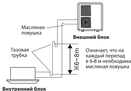
Наружный блок выше внутреннего
