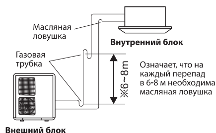
Наружный блок ниже внутреннего
